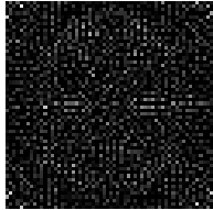
QR Zerlegung
