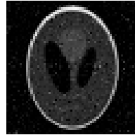
SVD
