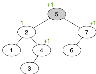
AVL-Baum
