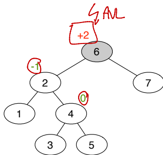
kein AVL-Baum!
