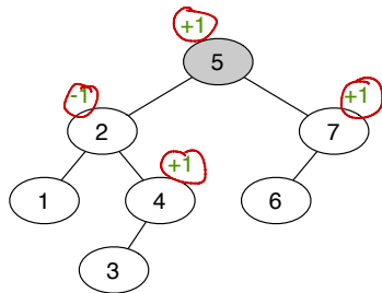
AVL-Baum
